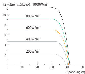
Strom-Spannung-Kurve (420W)
