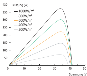
Leistung-Spannung-Kurve (420W)
